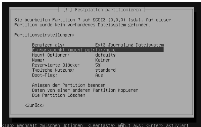
Abbildung 3.6: Datenpartition manuell einrichten
