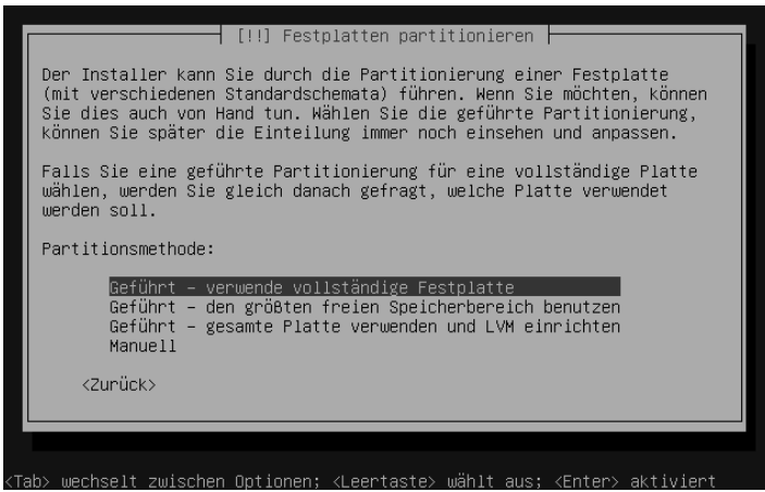
Abbildung 3.1: Partitionierung der Festplatte
