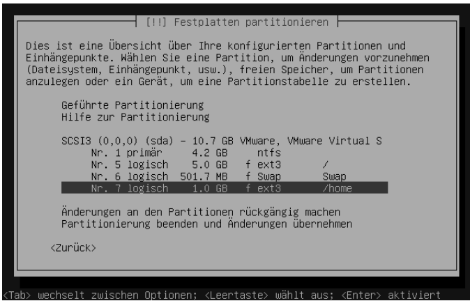
Abbildung 3.7: Die fertige Partitionstabelle
