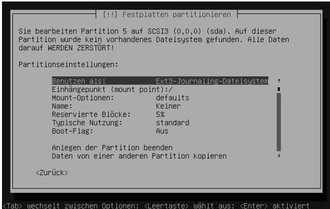
Abbildung 3.4: Systempartition manuell einrichten
