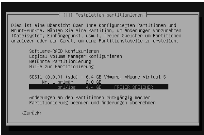
Abbildung 3.3: Die Partitionstabelle nach der Verkleinerung der Windows-Partition
