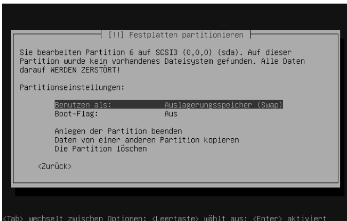
Abbildung 3.5: Swap-Partition manuell einrichten
